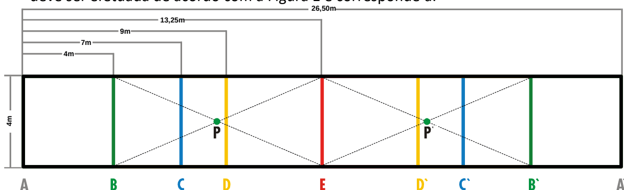
Figura 1: Configurações de cancha de bocha de 26,5m de comprimento e 4,0m de largura.
