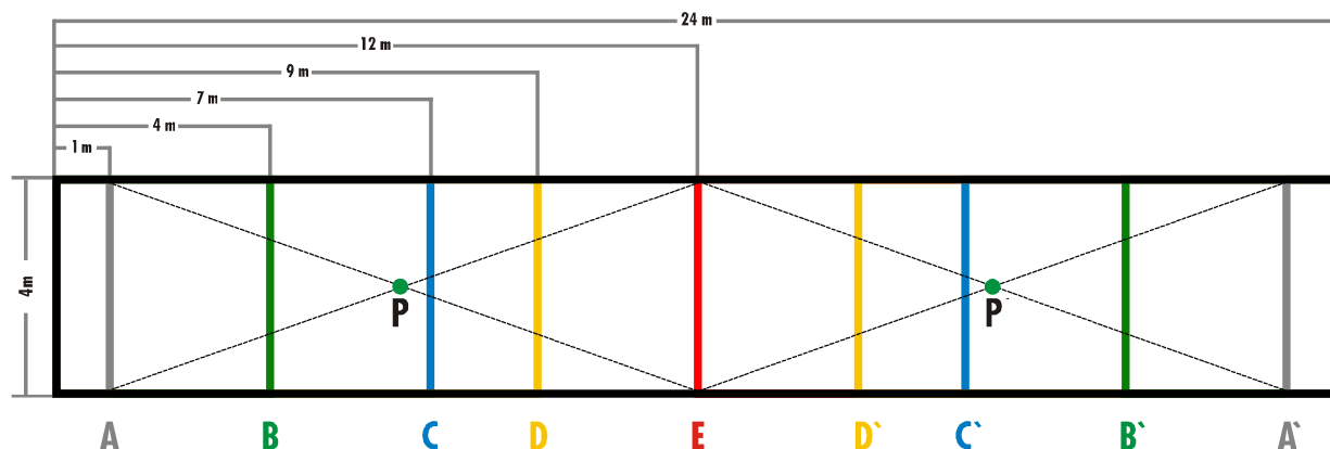
Figura 2: Configurações de cancha de bocha de 24,0m de comprimento e 4,0m de largura
